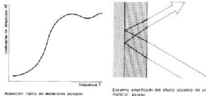
Absorción típica de materiales porosos poroso
